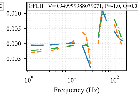
Re(Y dq )
