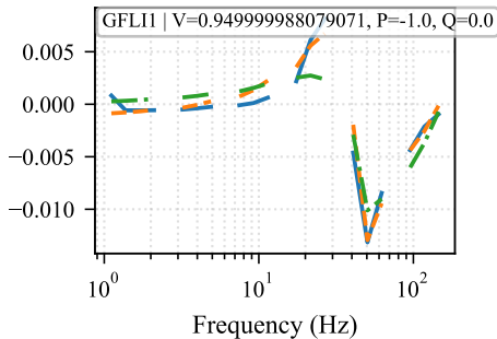
Re(Y qd )
