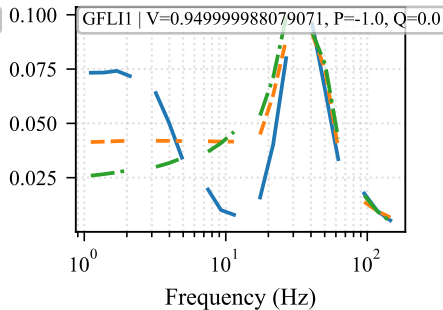
Re(Y qq )
