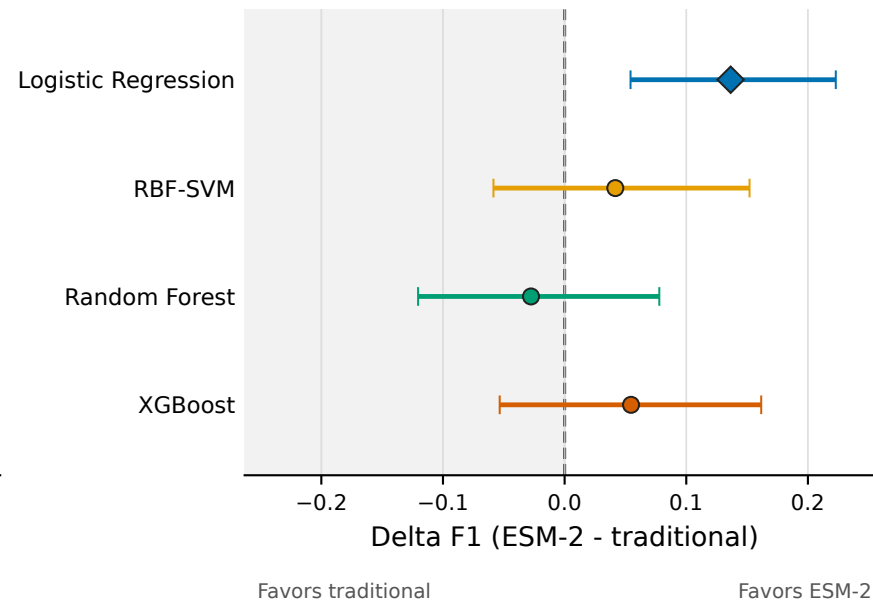
D F1
