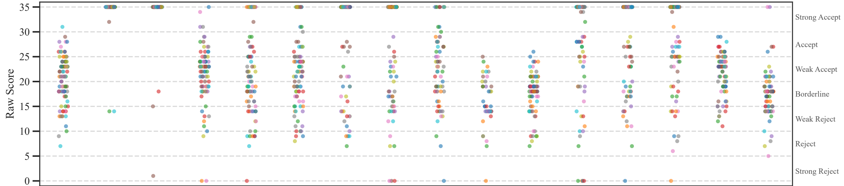
Model: mistral-small:22b
