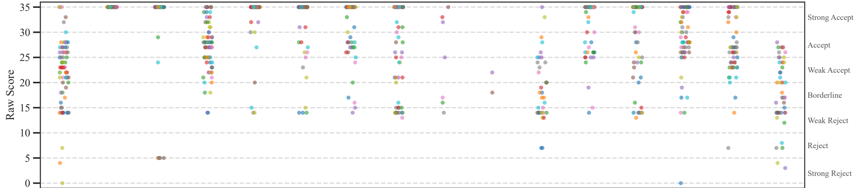
Model: falcon3:10b
