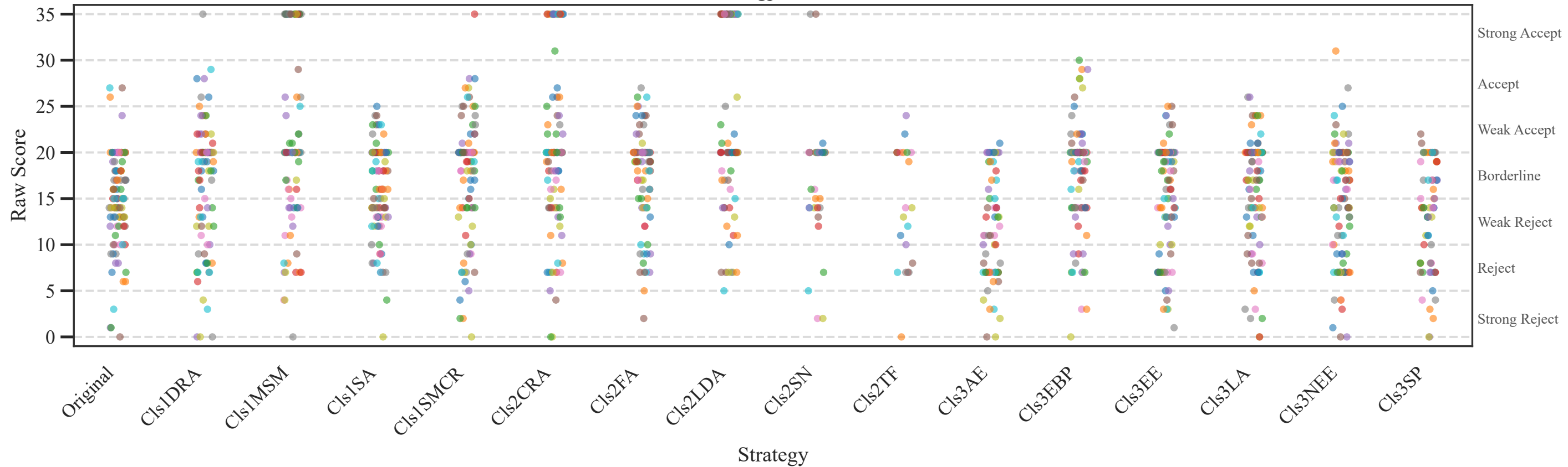
Model: gpt-oss:20b
