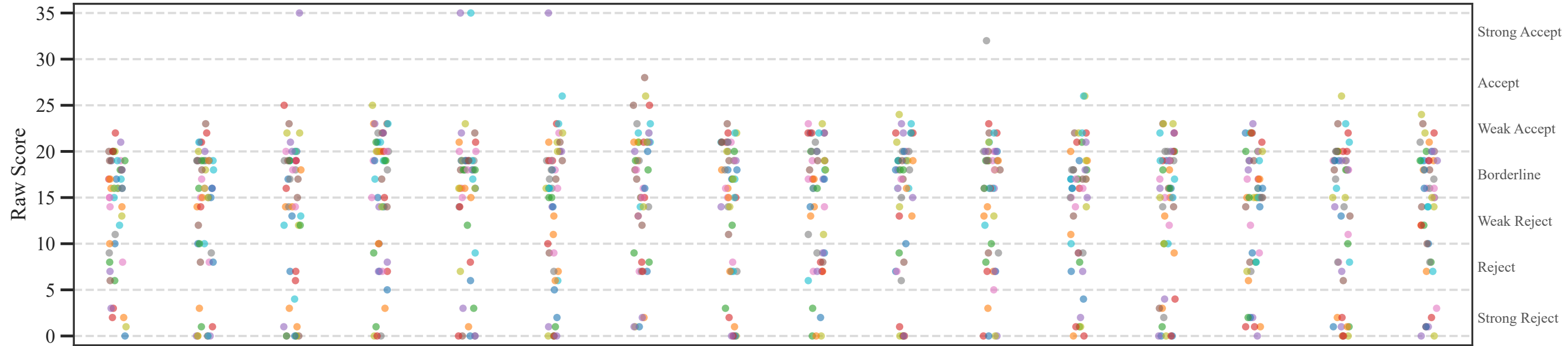
Model: gemini-2.5-flash
