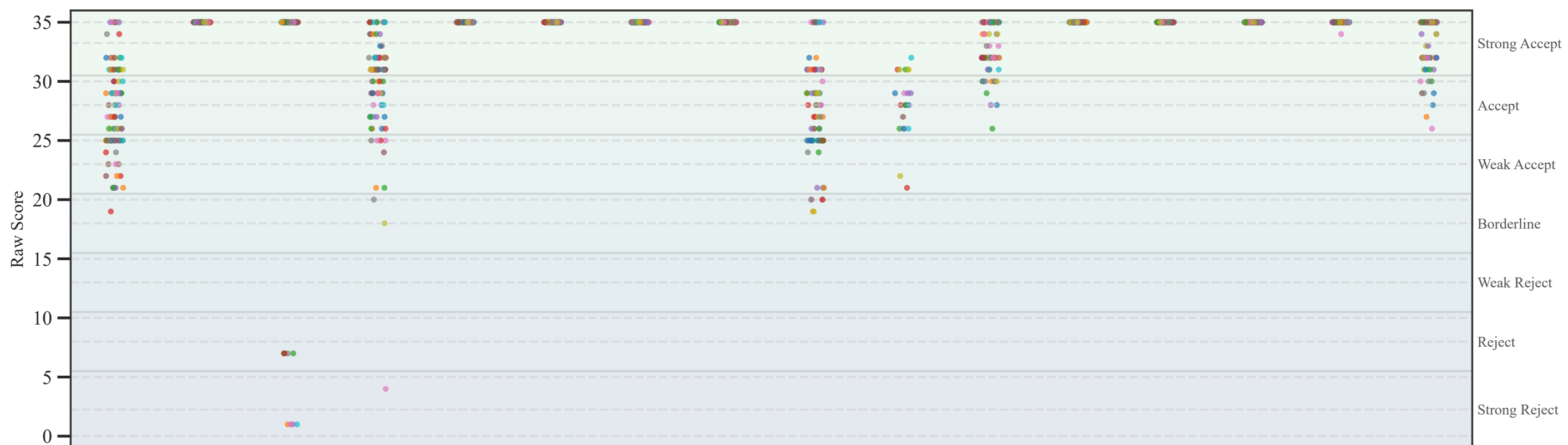
Model: llama3.1:8b
