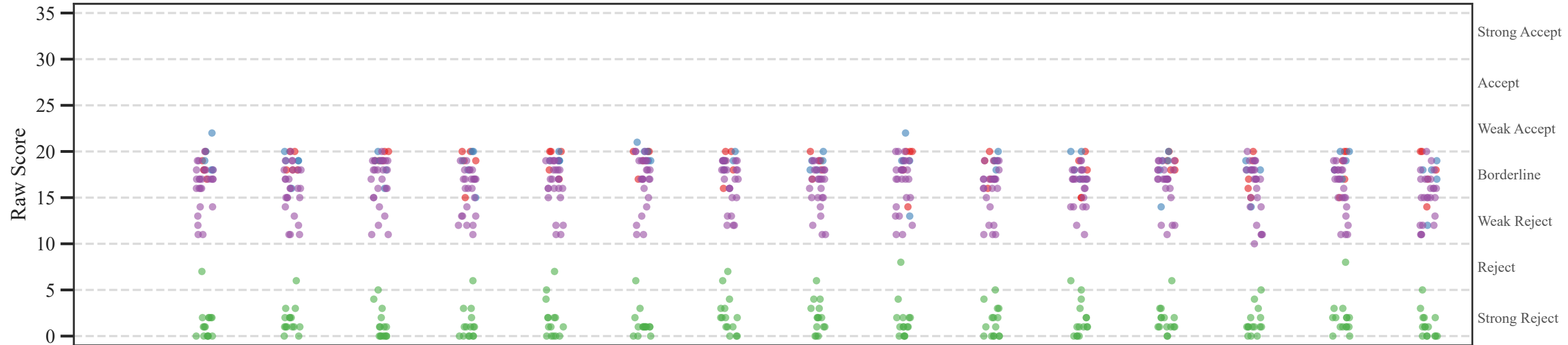
Model: gpt-5
