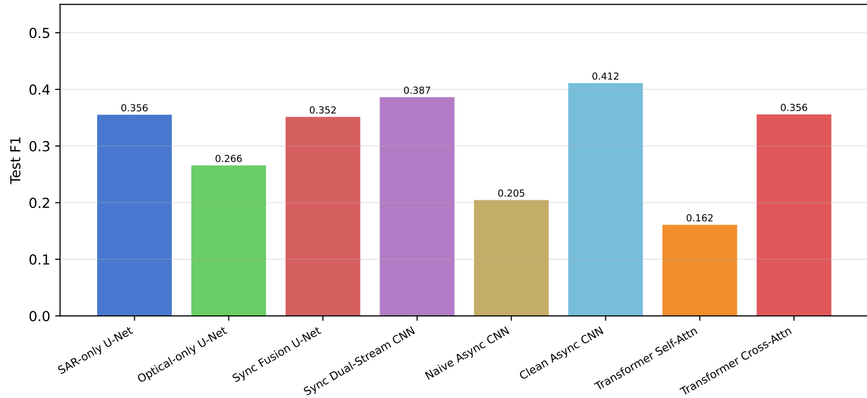
Test F1 by model
