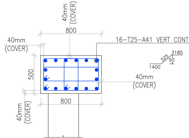
33 COLUMN C4 SCALE: 1:25
