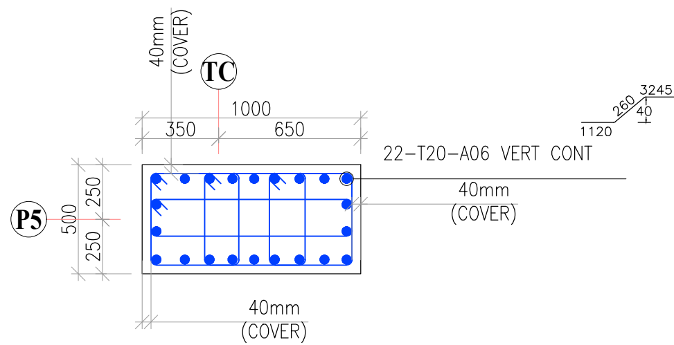
30 COLUMN C2 SCALE: 1:25
