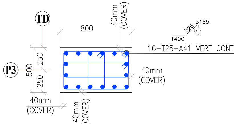
31 COLUMN C4 SCALE: 1:25
