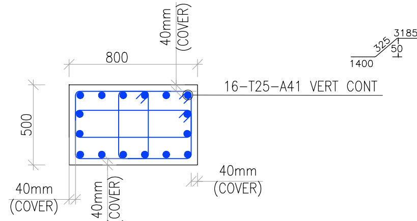
32 COLUMN C4 SCALE: 1:25
