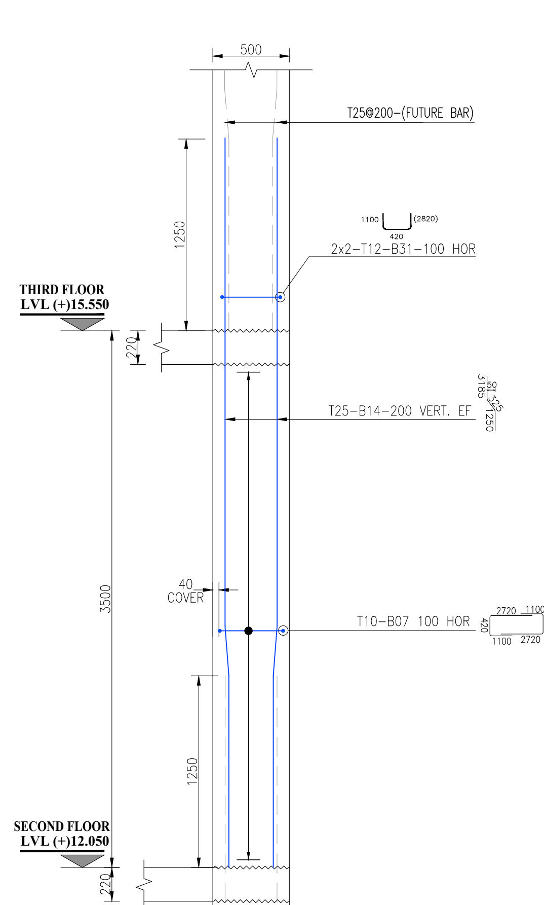
SECTION-2A SCALE: 1:25
