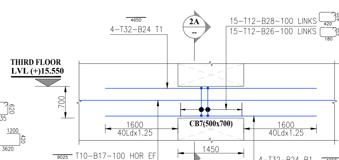
DETAIL-2 SCALE: 1:50
