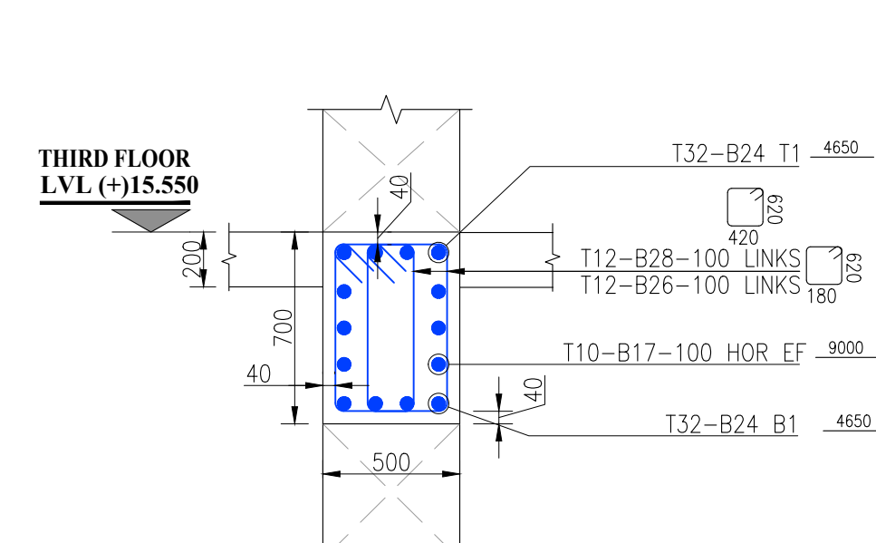
SECTION-2A SCALE: 1:25
