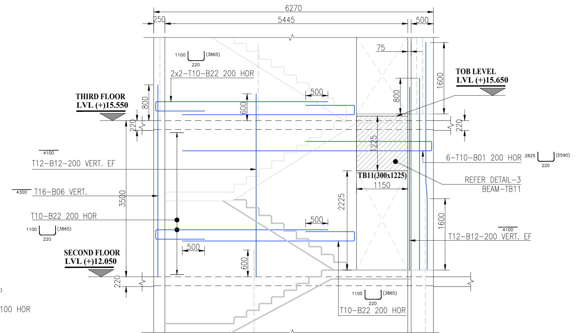
ELEVATION-B SCALE: 1:50
