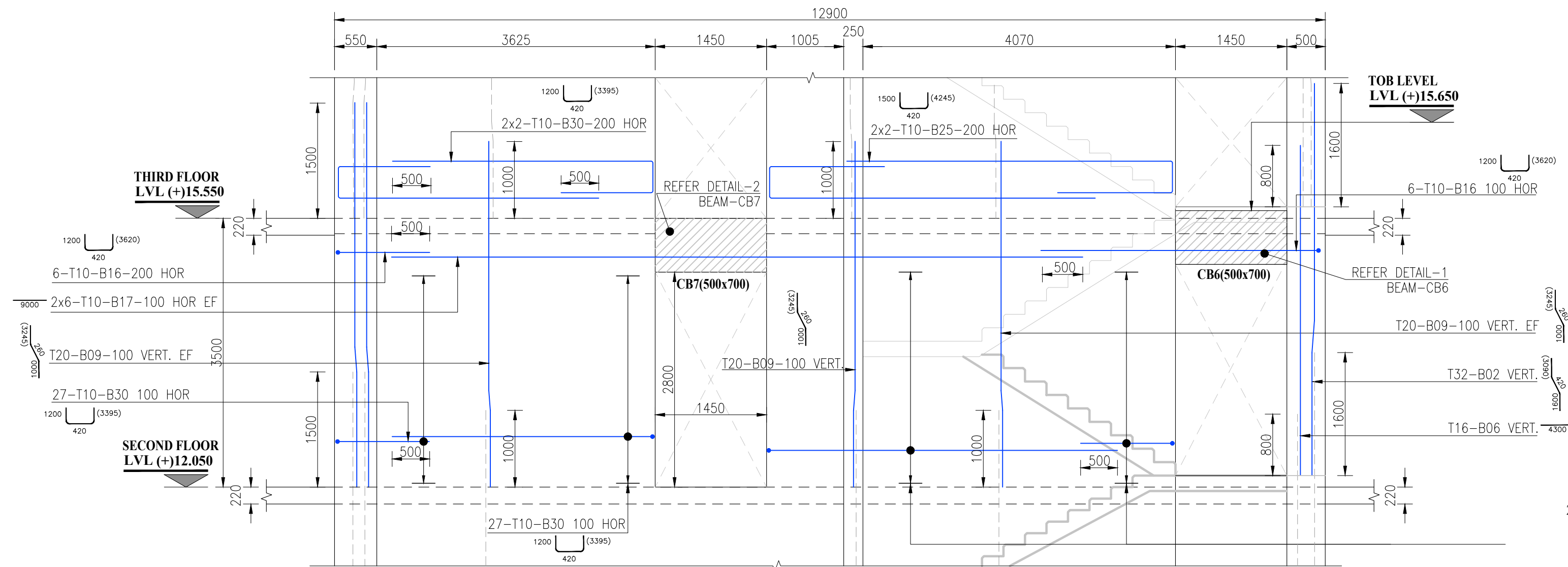
ELEVATION-A SCALE: 1:50
