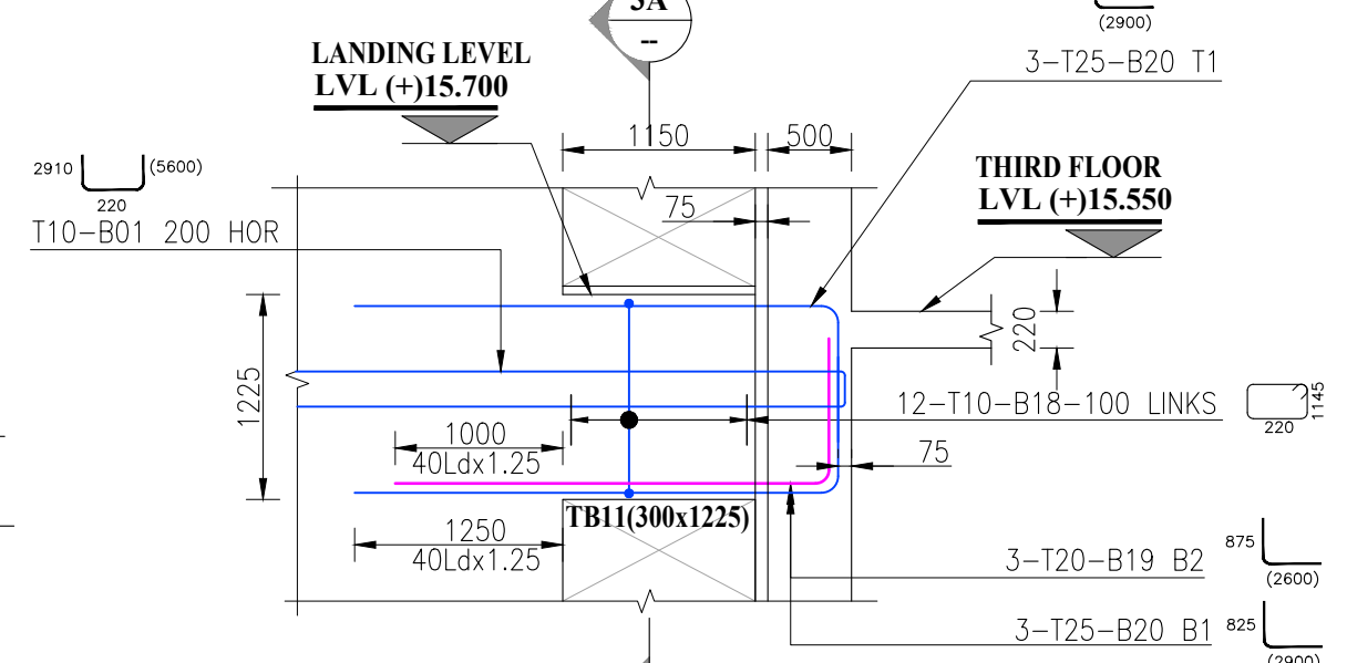
DETAIL-3 SCALE: 1:50
