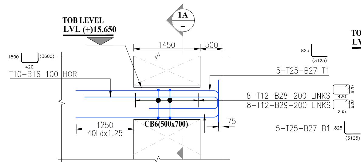
DETAIL-1 SCALE: 1:50
