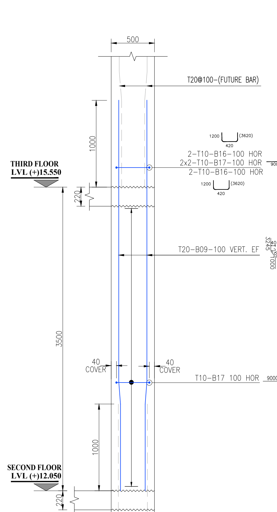
SECTION-2 SCALE: 1:25
