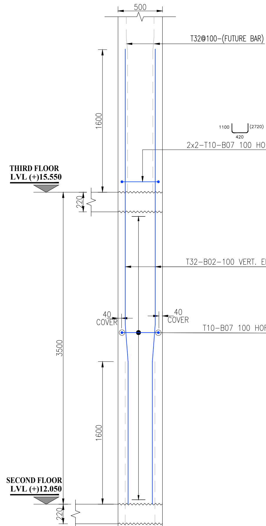
SECTION-1 SCALE: 1:25
