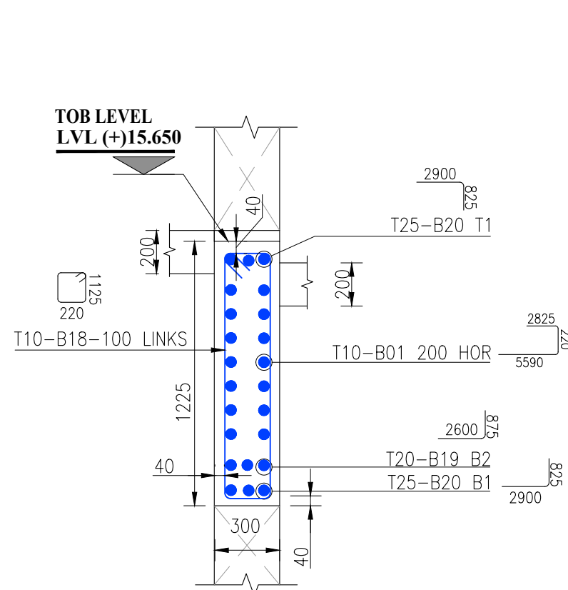
SECTION-3A SCALE: 1:25
