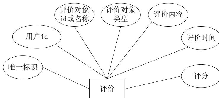
图 4.14 评价实体图
