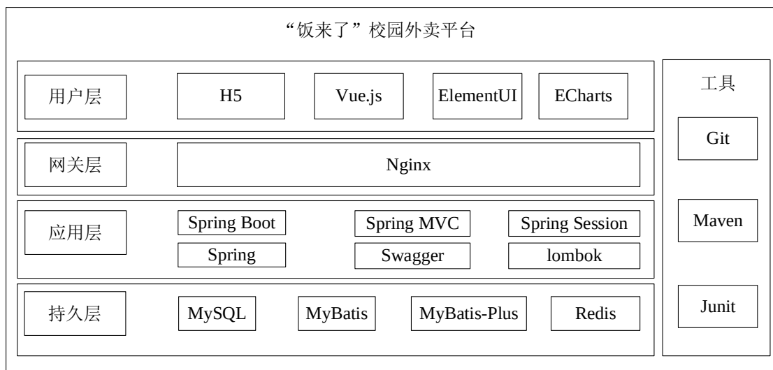
图 4.1 总体架构图
