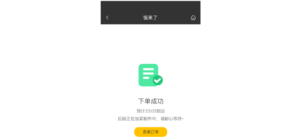
图 6.7 测试成功图
