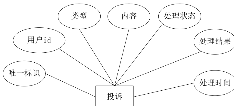
图 4.15 投诉实体图
