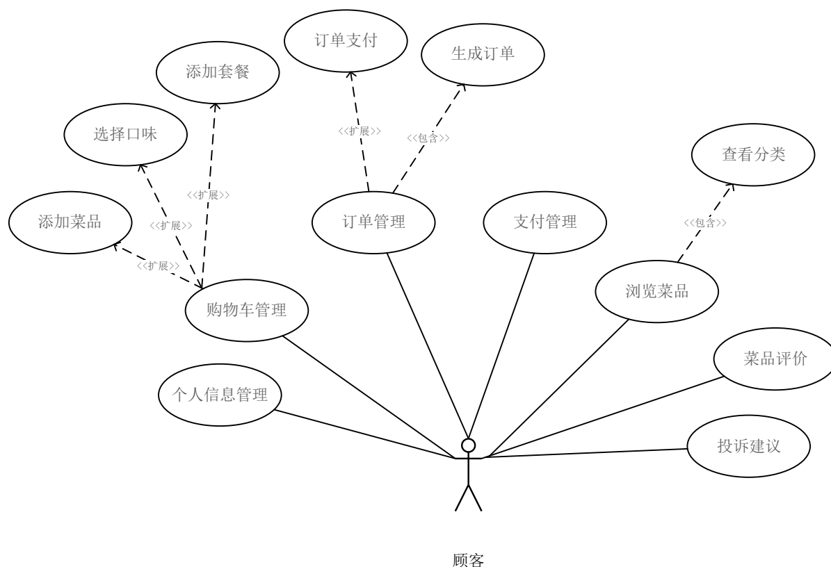
图 3.1 顾客用例图
