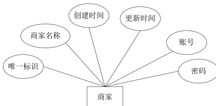
图 4.16 商家实体图
