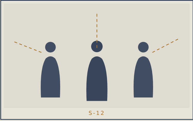
S-12
