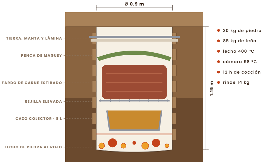
Corte axial del horno, levantado a escala de la ficha del chef
