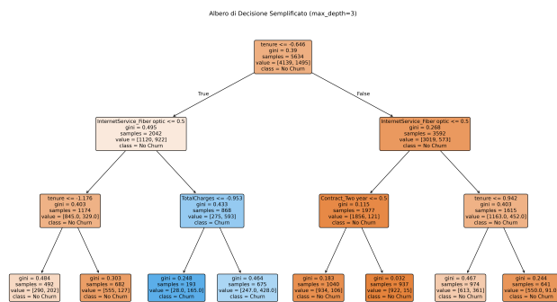
Figura 4: Albero di Decisione semplificato ( max\_depth = 3 ).
