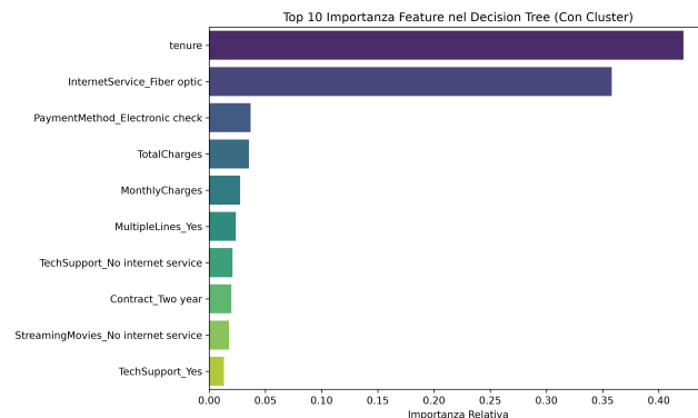
Figura 5: Top 10 importanza delle feature nello Scenario B.
