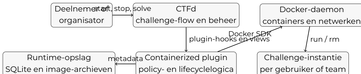
Figuur 6.1: Architectuur van de plugin-PoC. CTFd blijft het centrale platform, terwijl de plugin de lifecycle van challenge-containers en de bijhorende metadata beheert. De Docker-daemon kan lokaal of op een afzonderlijke runtime-host draaien.
