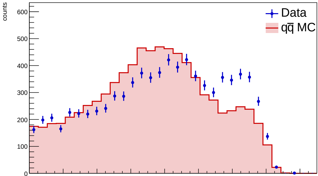
Zernike Moment 51
