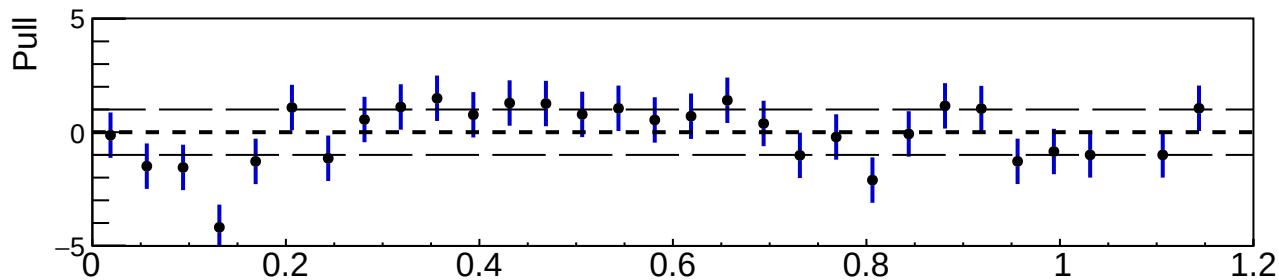
Zernike Moment 51
