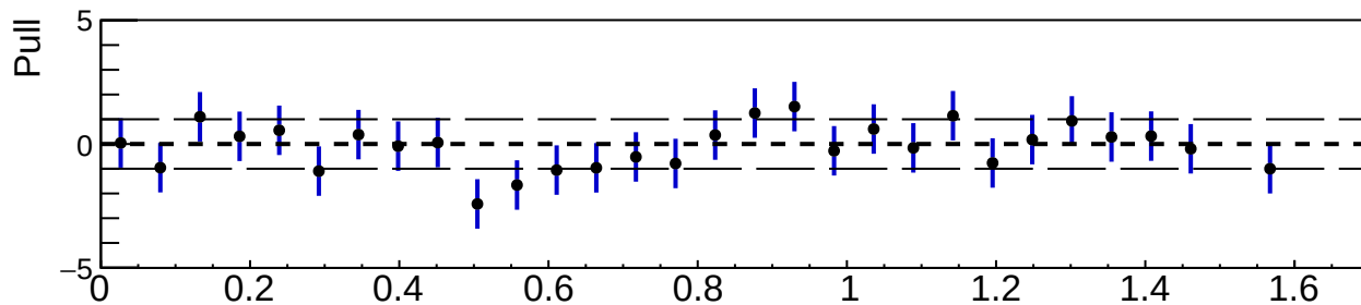
Zernike Moment 51
