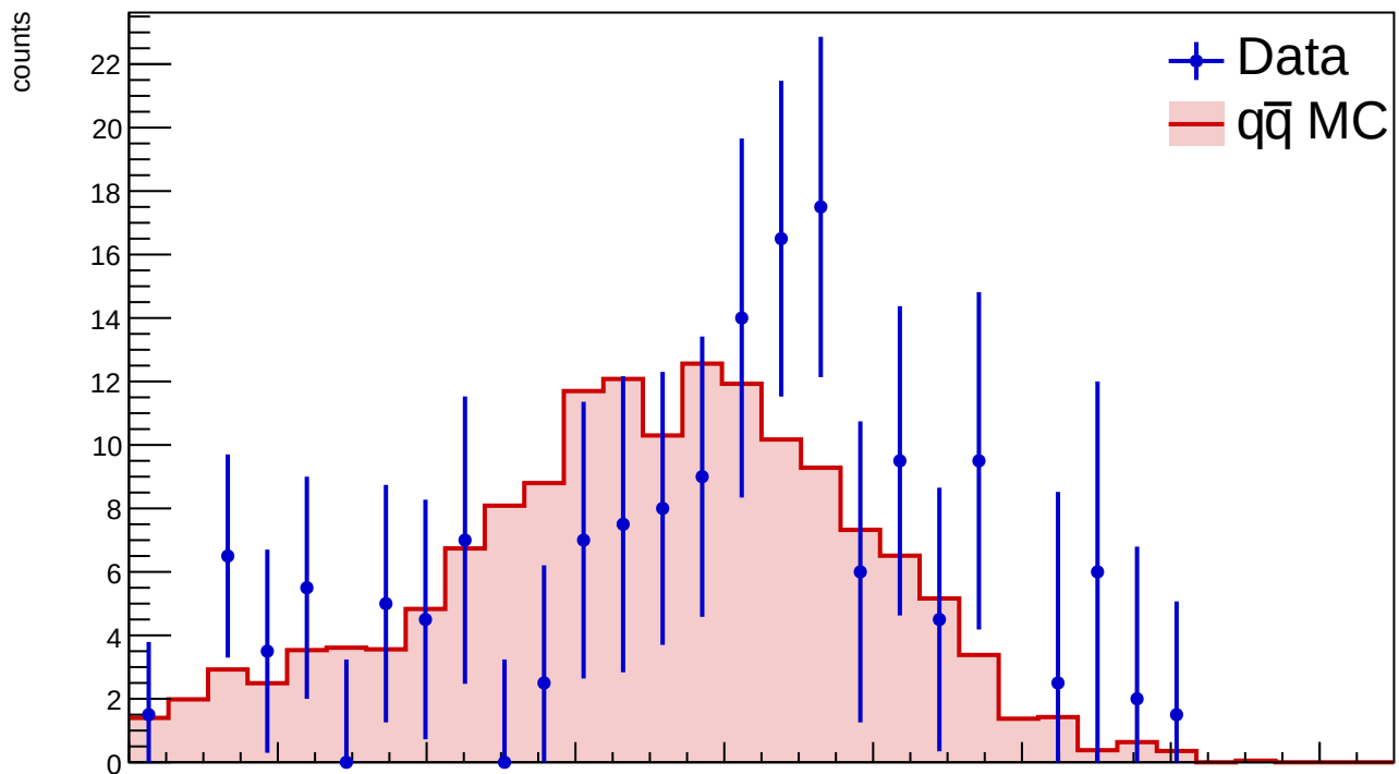
Zernike Moment 51
