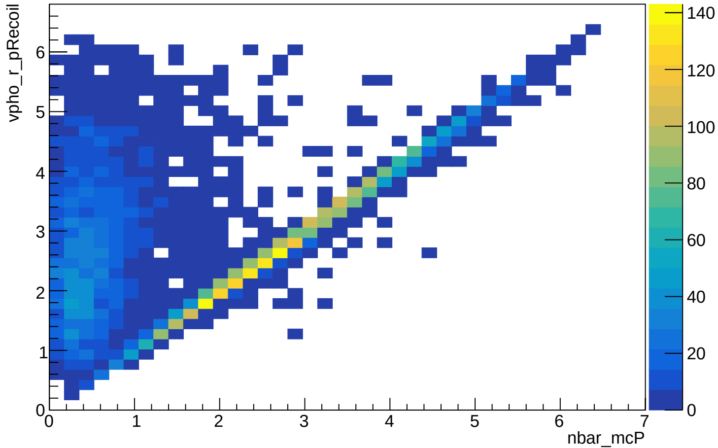
vpho_r_pRecoil:nbar_mcP
