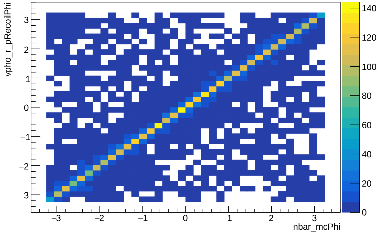
vpho_r_pRecoilPhi:nbar_mcPhi
