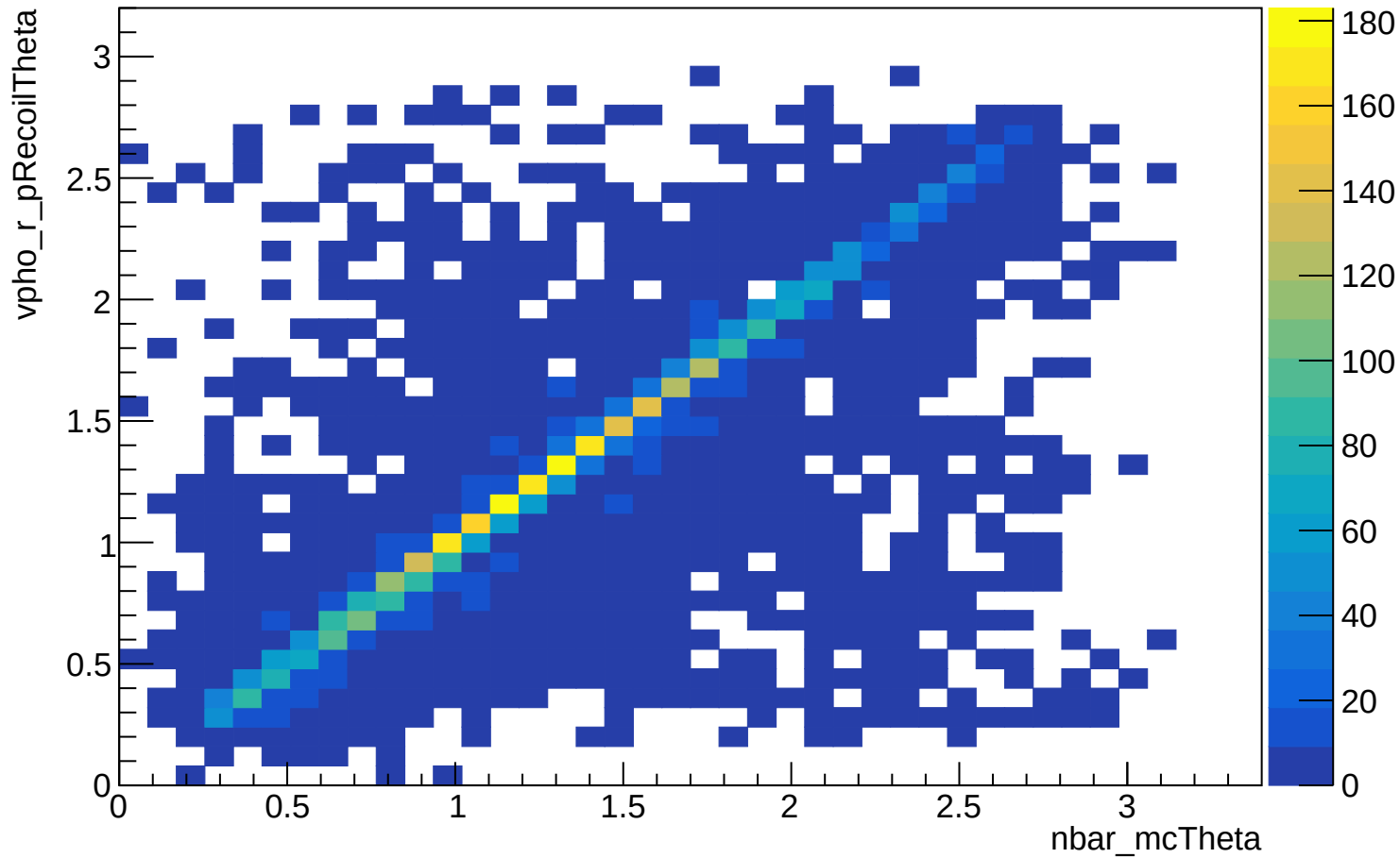
vpho_r_pRecoilTheta:nbar_mcTheta
