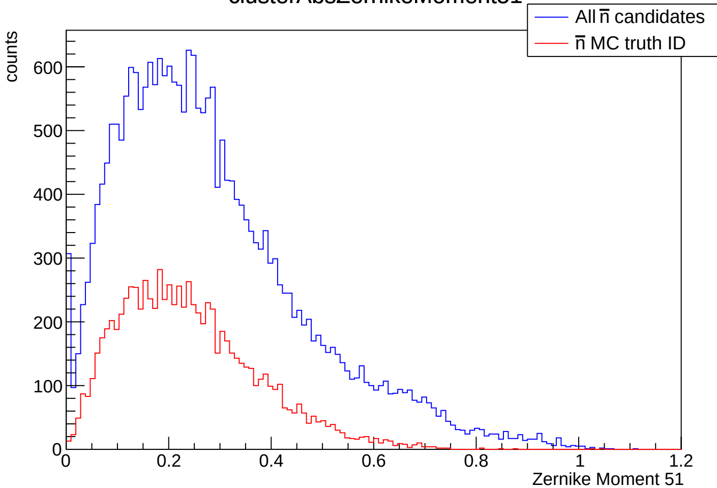
clusterAbsZernikeMoment51
