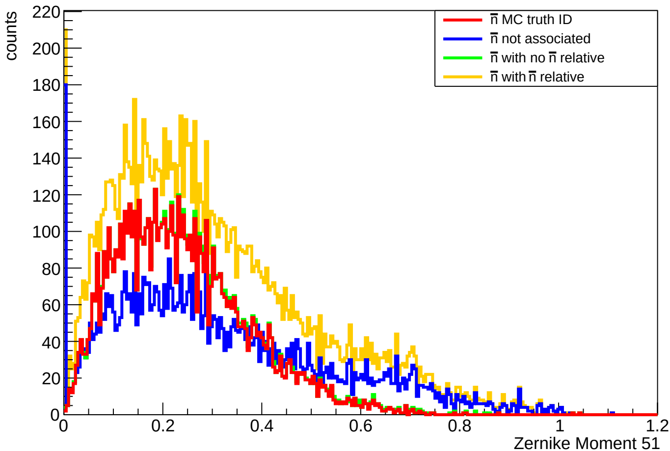
clusterAbsZernikeMoment51
