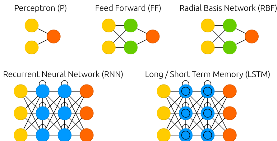
Figura 3.2: Esquema de topologías básicas de redes neuronales, desde el perceptrón hasta arquitecturas con capas ocultas y conexiones recurrentes [11].
