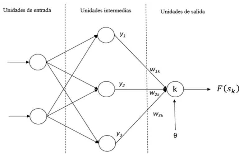
Figura 3.1: Esquema de una red neuronal simple. [10]
