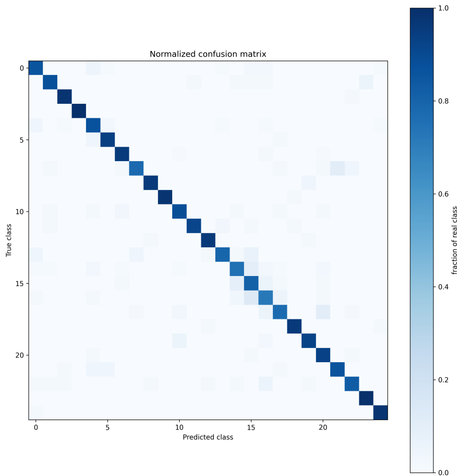
Figura 4.2: Matriz de confusion obtenida experimentalmente utilizando el modelo Hybrid-CustomTTN
