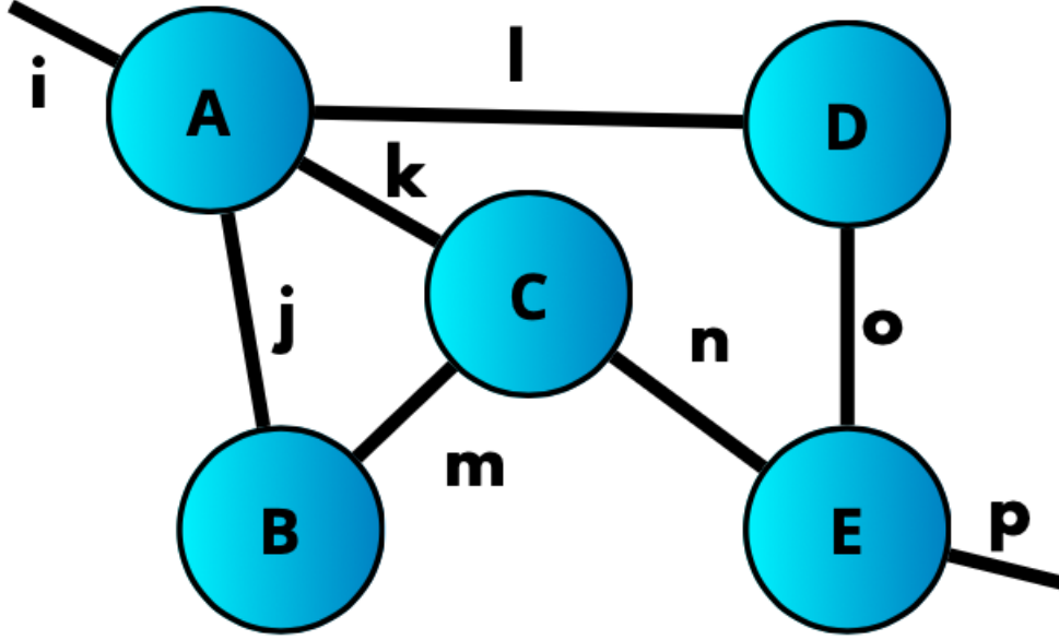
Figura 3.4: Ejemplo de representación diagramática para un tensor. Fuente: [14]
