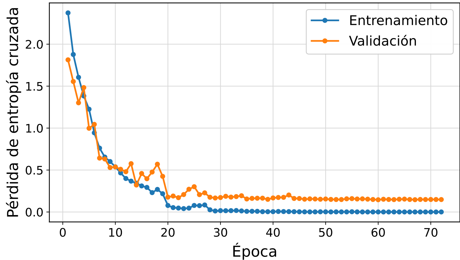
Pérdida de ResNet50 (desde cero)
