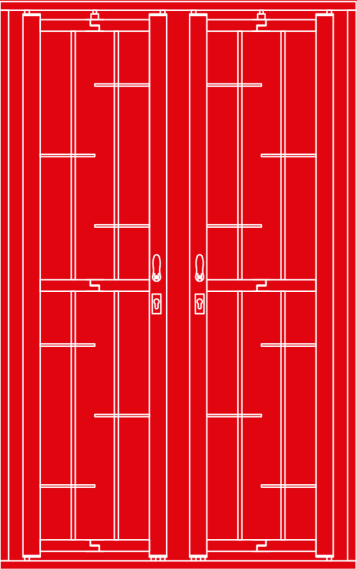
Mod. E - Tondino diam. 14 verticale - Piatto orizzontale 30x8
