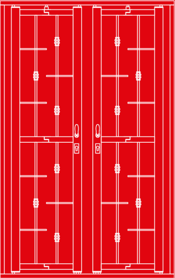
Mod. D - Tondino diam. 14 verticale - Piatto orizzontale 30x8 + borchie
