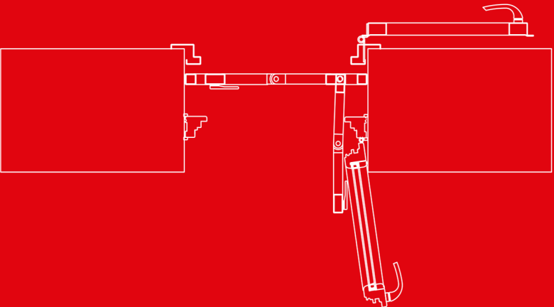
Grata interposta a snodo - apertura verso interno
