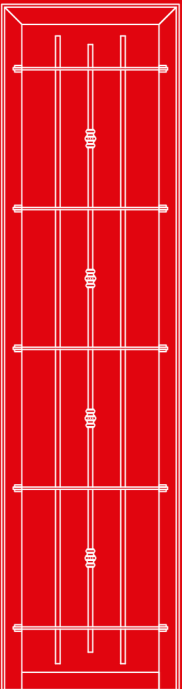
Mod. 3 - tondo diam. 14 - piatto 30x8 + mezzi cerchi
