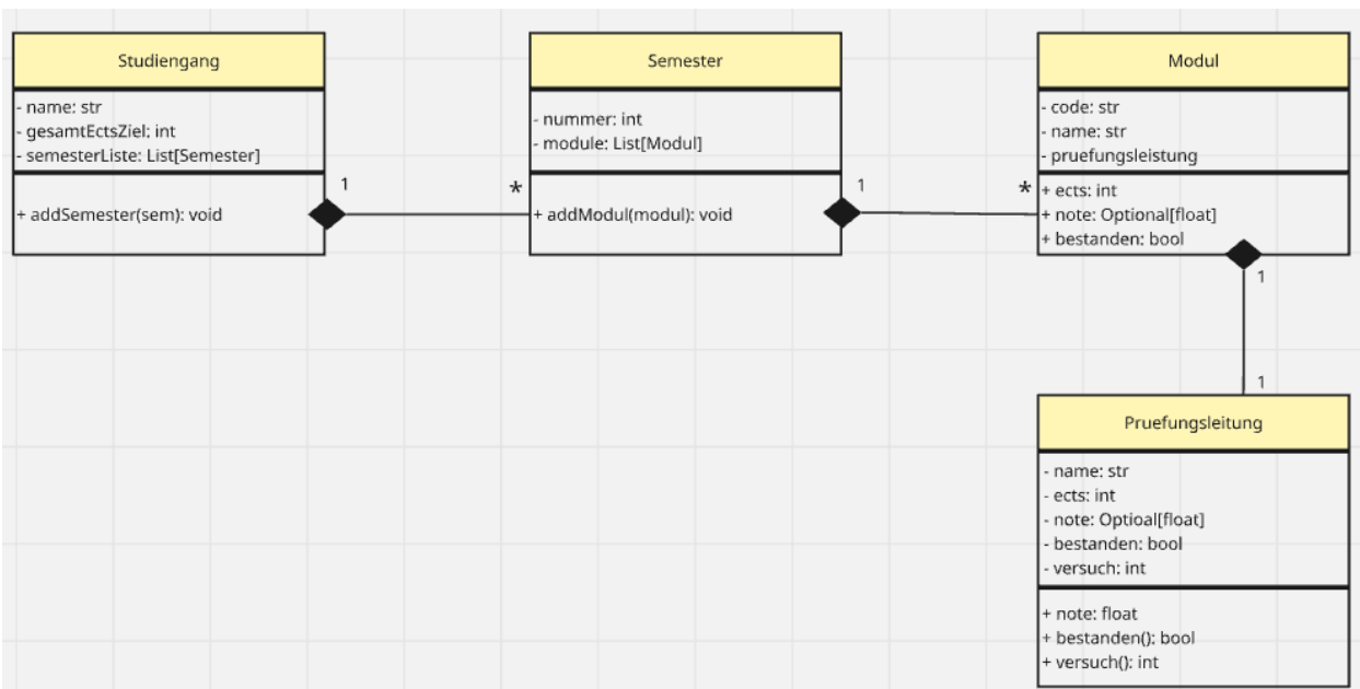
Abbildung 2: Plattformunabhängiges Entity-UML-Klassendiagramm (Konzeptionsphase)
