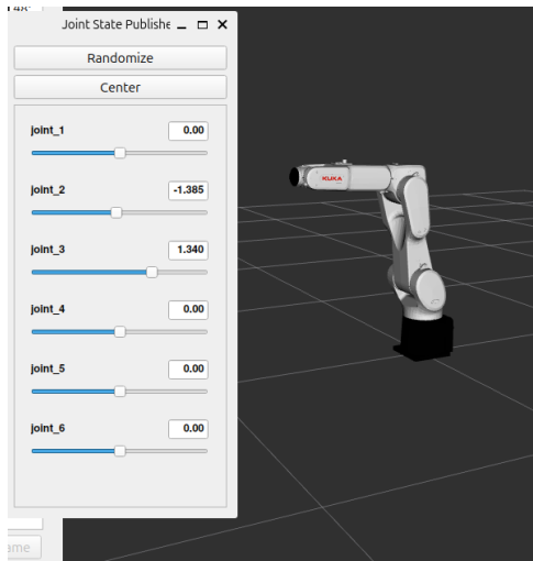
Figura 4. Evidencia de ejecución: Joint State Publisher GUI con las seis articulaciones y el modelo KUKA visualizado en RViz2.
