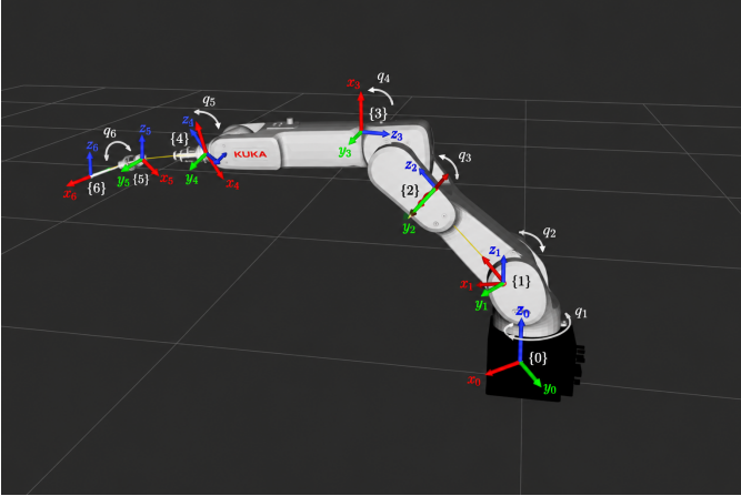
Figura 3. Asignación propia de marcos Denavit–Hartenberg utilizada en el modelo cinemático del KUKA KR 7 R900-3.
