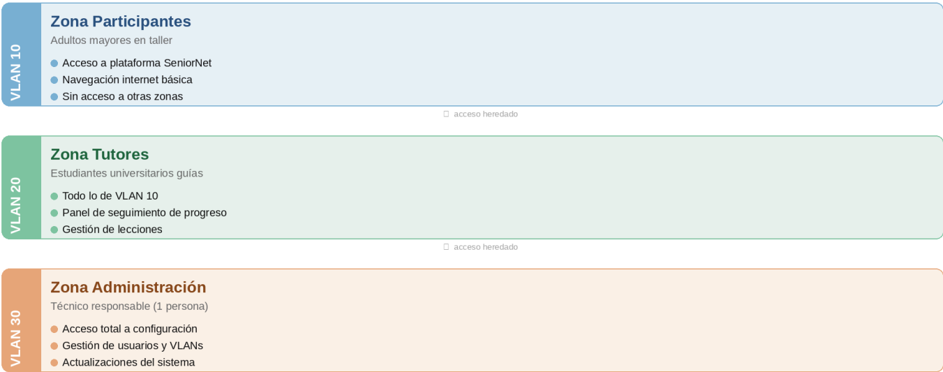
Figura 2 — Segmentación por VLANs: cada zona accede solo a lo que le corresponde
