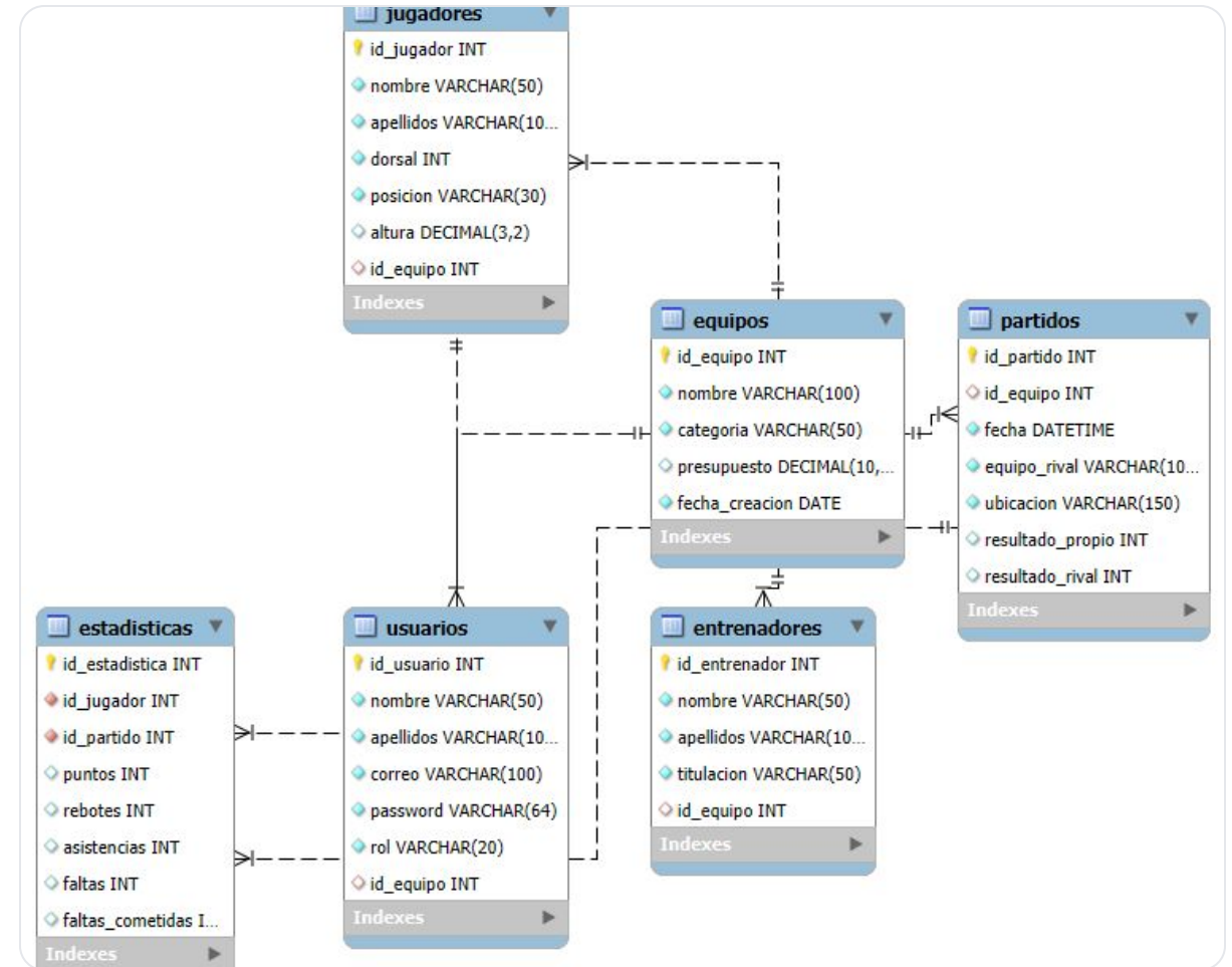
Diagrama de Entidad-Relación de la Base de Datos
