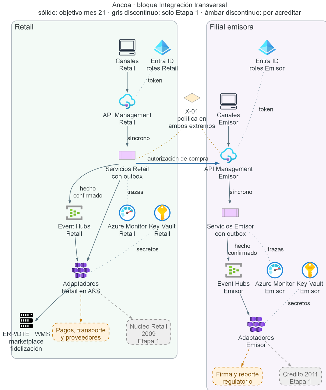
Figura 4.9: Bloque de integración. Fuente: elaboración propia a partir de SD-03 y RT-02.
