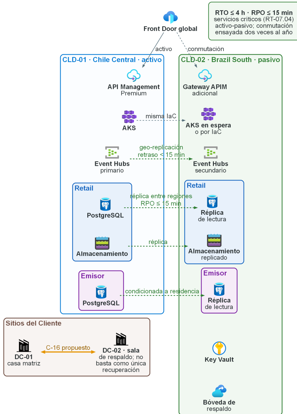
Figura 4.19: Centro de datos secundario y conmutación. Fuente: elaboración propia a partir de RT-03, RT-07 y SD-03.
