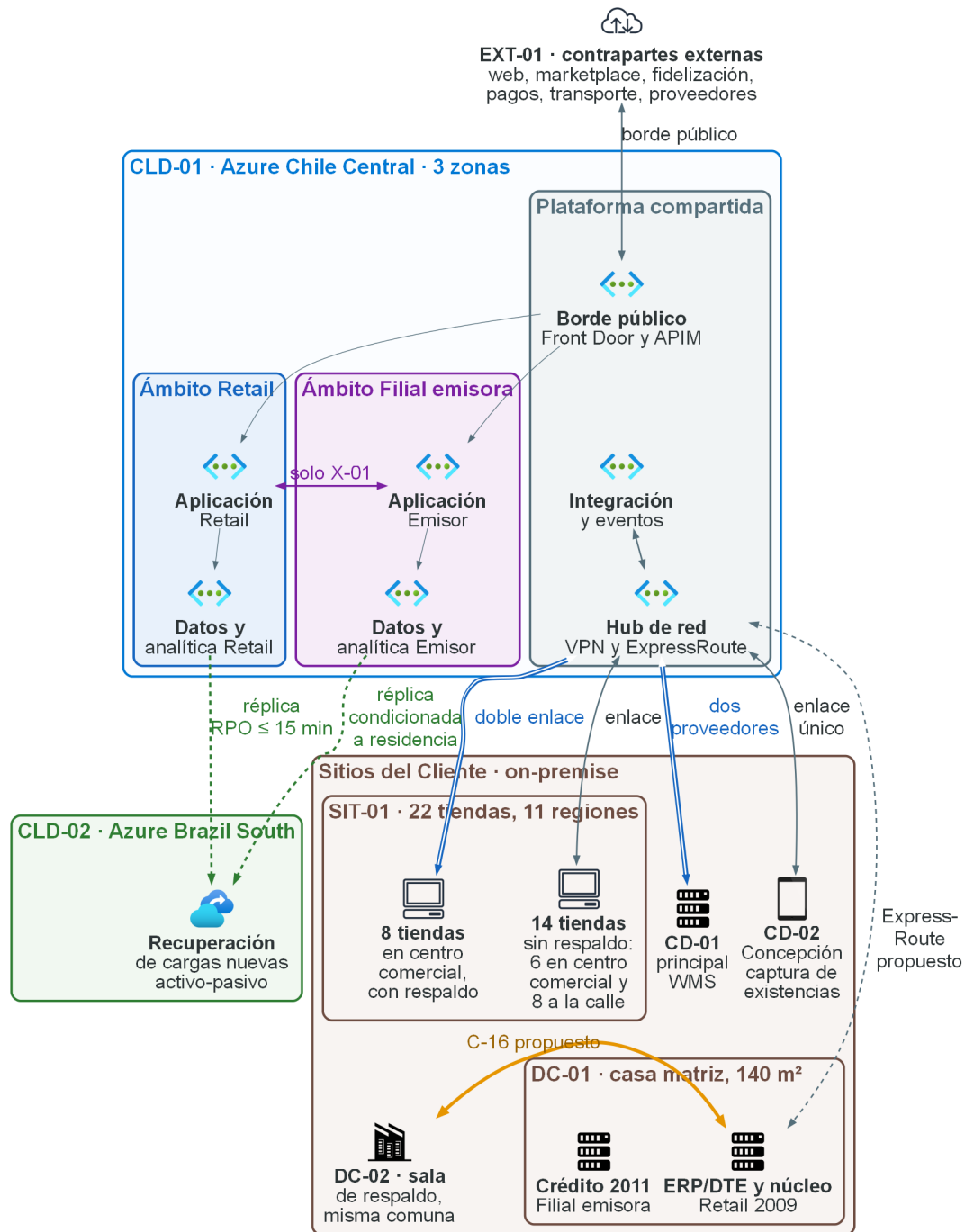
Figura 4.13: Arquitectura física general y emplazamiento de los sitios. Fuente: elaboración propia a partir del Caso 09, RT-03 y SD-03.
