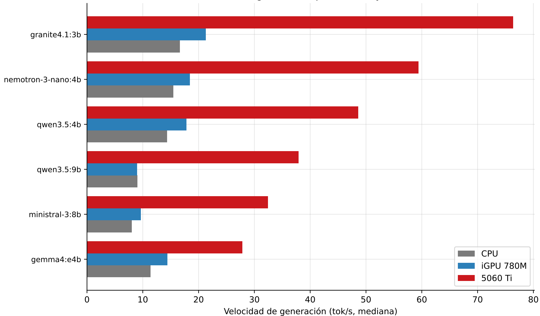
Velocidad de generación por modelo y hardware
