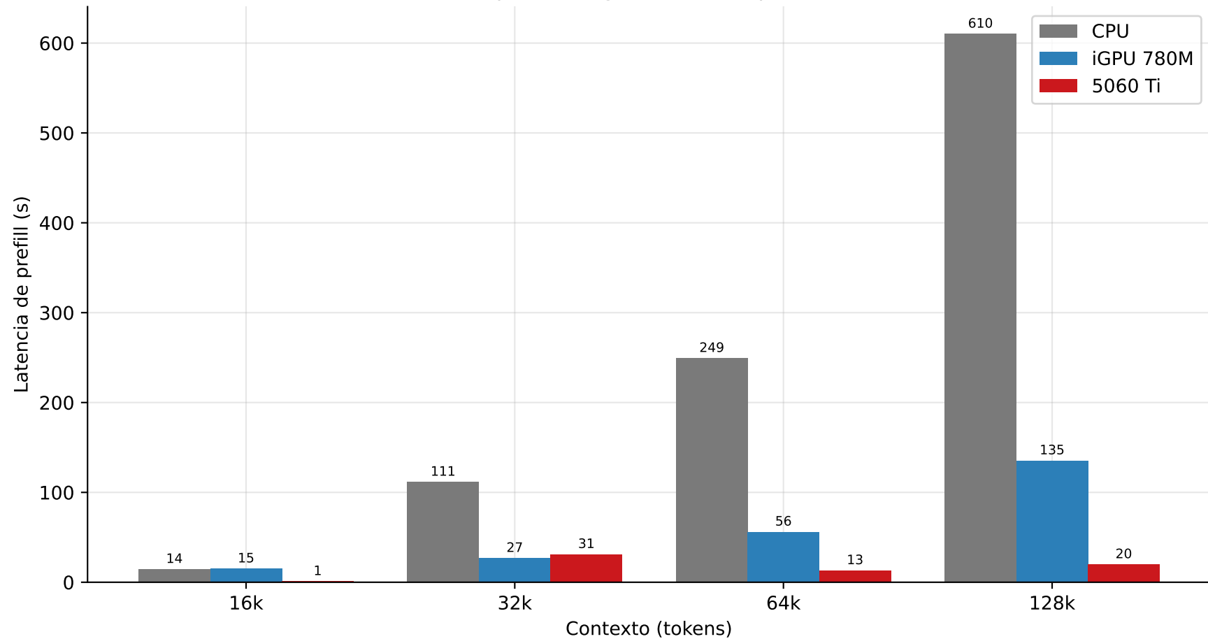
Coste de prefill de gemma4:e4b por hardware
