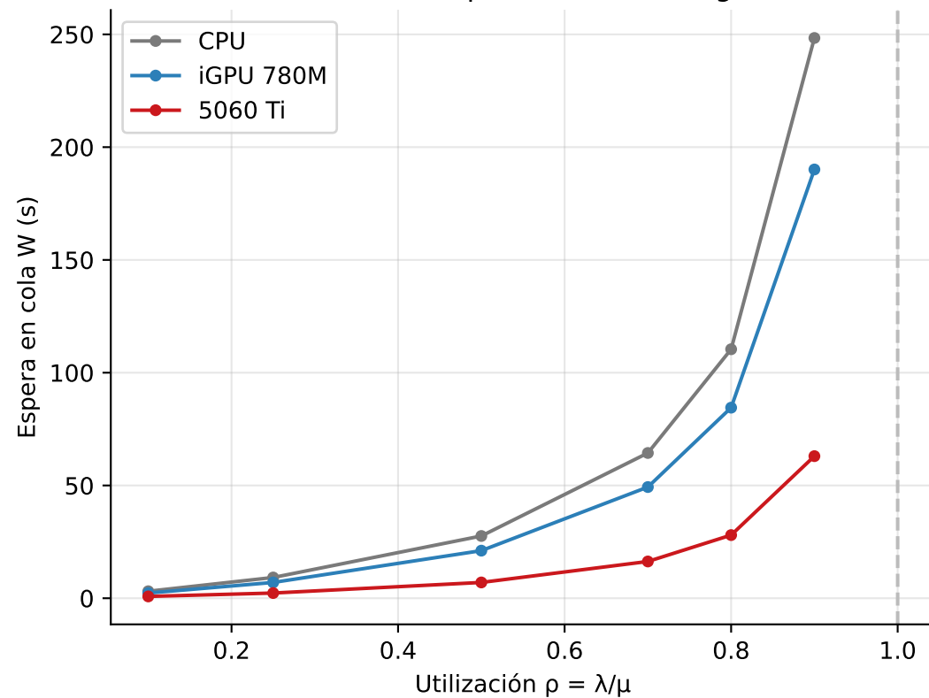
M/M/1: la espera a misma carga
