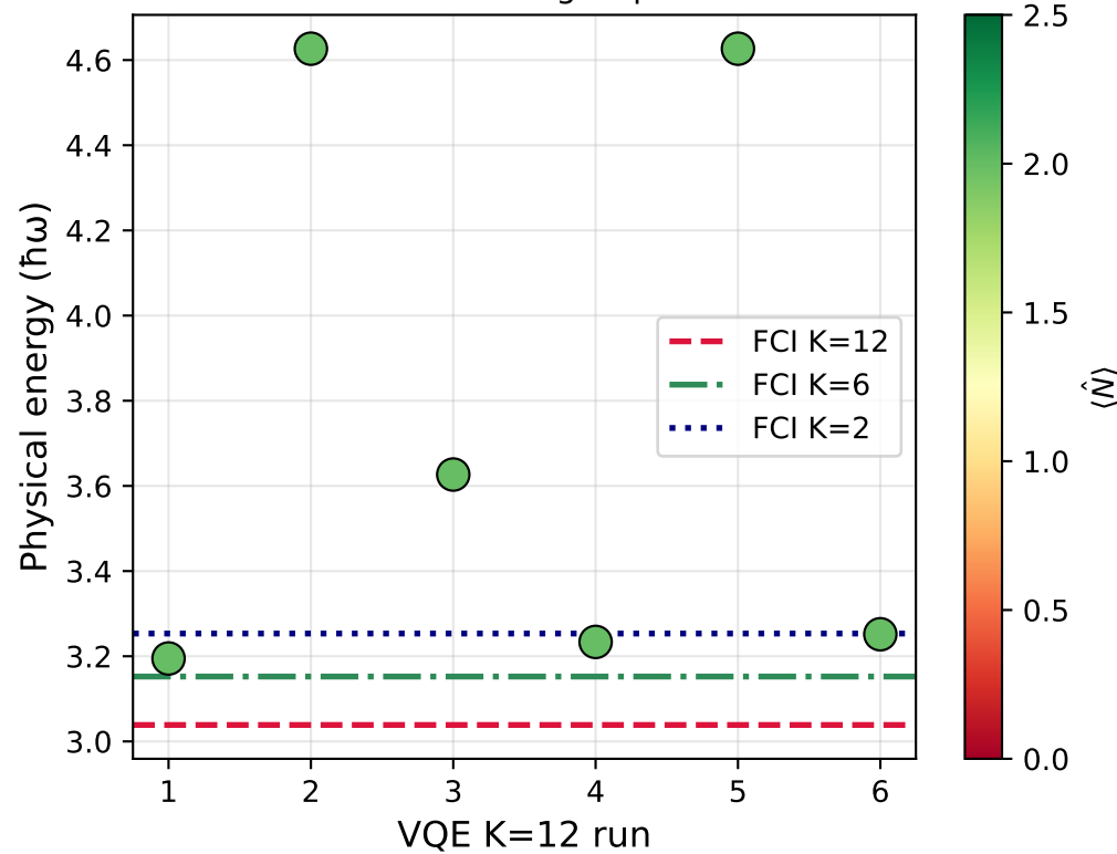
Final K=12 energies per run
