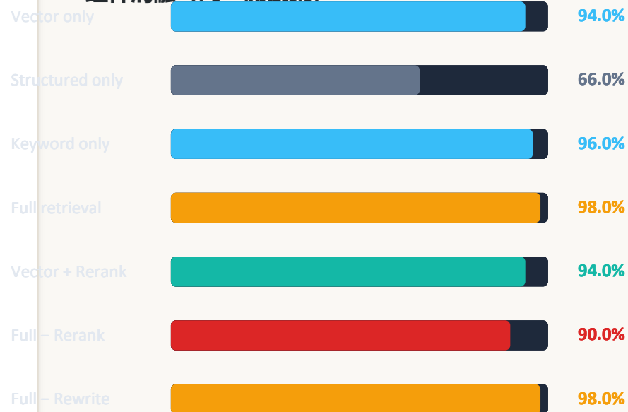
7 组受控消融 (同一 50 题测试集) 组件消融 (同一测试集)
