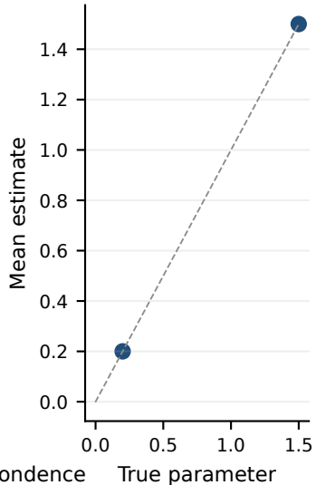
Parameter recovery
