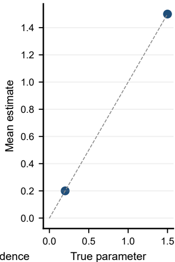
Parameter recovery
