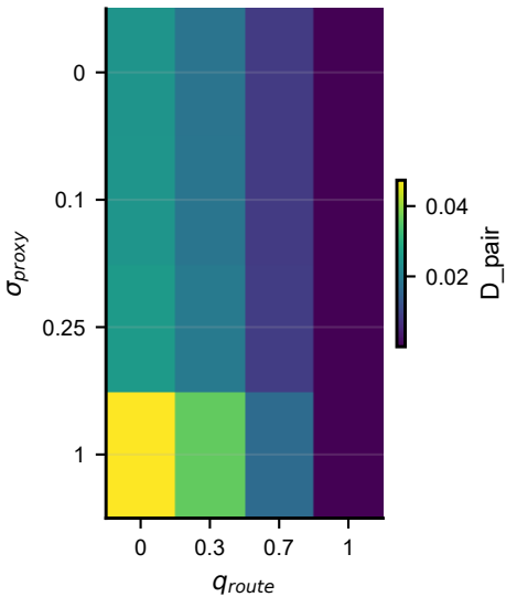
D_pair heatmap
