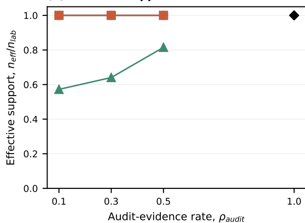
(d) Effective support
