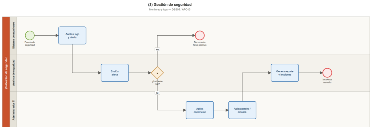
Diagrama BPMN 2.0 — Proceso 3: Gestión de seguridad.
