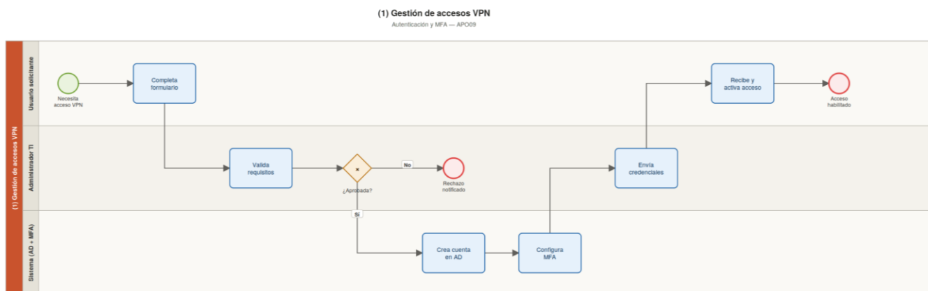
Diagrama BPMN 2.0 — Proceso 1: Gestión de accesos VPN.
