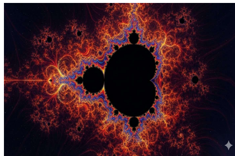
Conjunto de Mandelbrot
