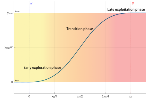
图4. S形 \text{optRatio}(t) 关于迭代次数的曲线图。
