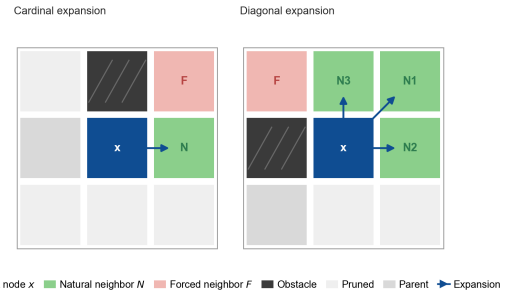
图 1. JPS邻居剪枝规则示意图。
