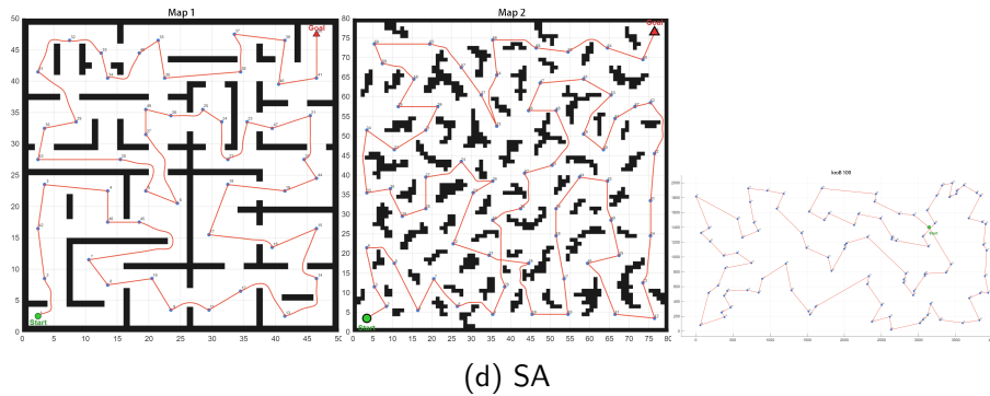
图 19. 每个旅行商求解器在三张地图上规划的最优代价值路径。每行从左至右依次为 Map 1、Map 2、Map 3。
