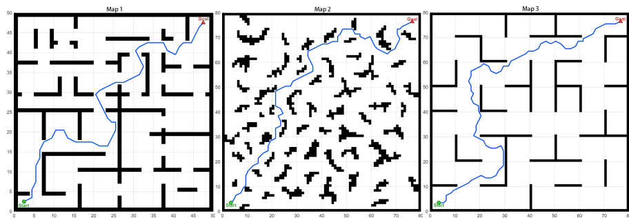
(d) RRT
