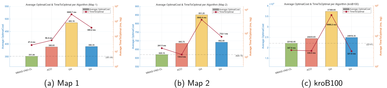
图 18. 四个旅行商求解器在三张地图上的平均代价与平均计算时间对比。
