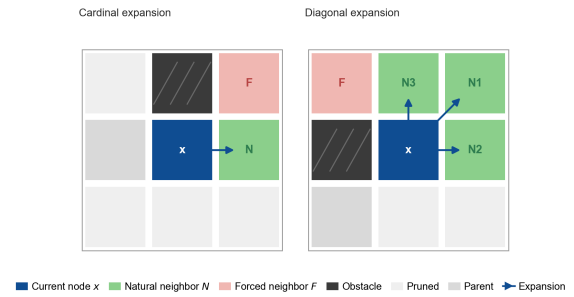
图 1. JPS 邻居剪枝规则示意图。
