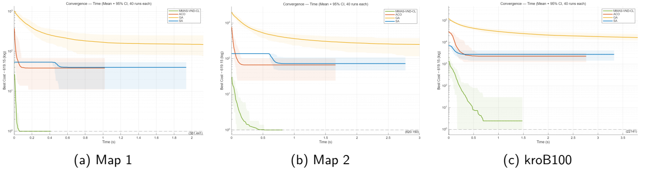
图 16. 四个旅行商求解器在三张地图上 40 次运行的平均时间-代价收敛曲线。
