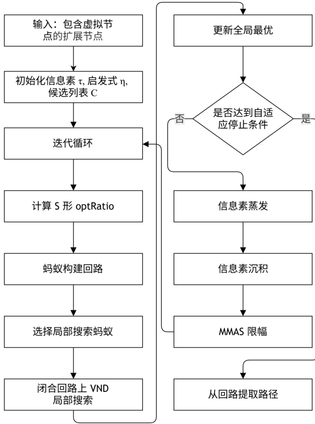
图 5. 改进蚁群优化总体流程图。
