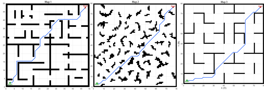
(c) Dijkstra
