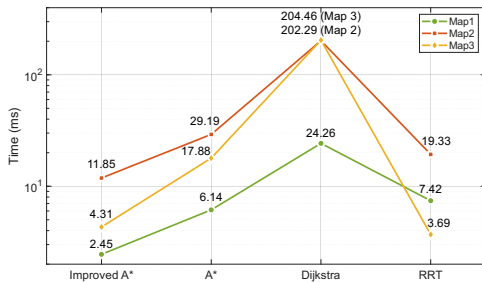
图 9. 四个算法在Map 1、2、3上的计算时间对比（折线图）。
