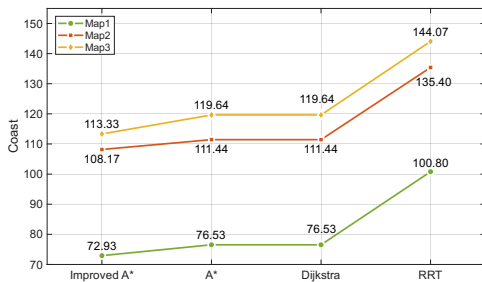
图 8. 四个算法在Map 1、2、3上的路径长度对比（折线图）。
