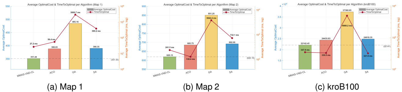
图 17. 四个旅行商求解器在三张地图上的平均代价与平均计算时间对比。
