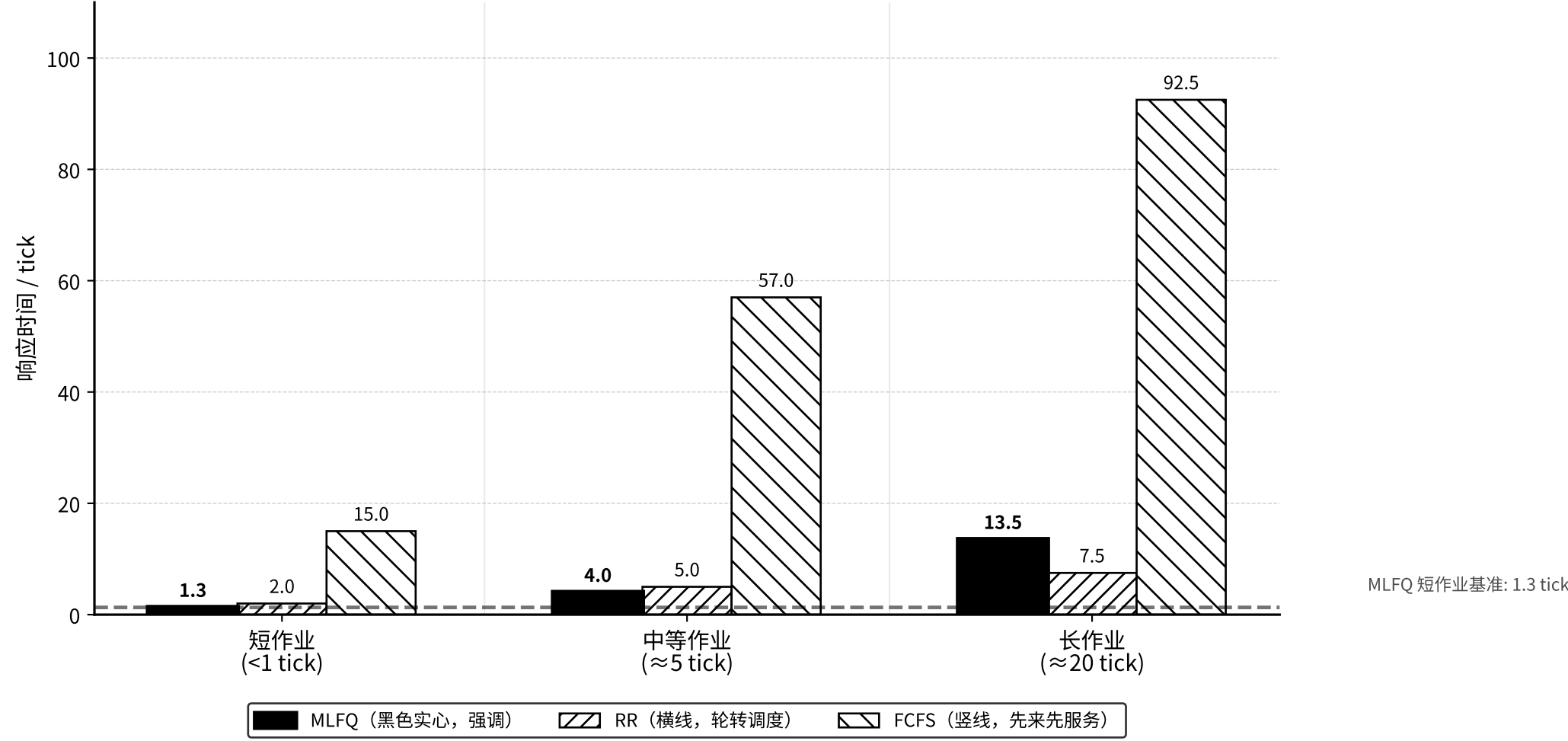
图 S4-1 MLFQ / RR / FCFS 调度算法响应时间对比
