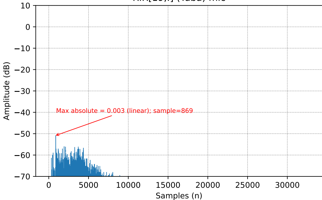
RIR[19,:] (Tuba) mic
