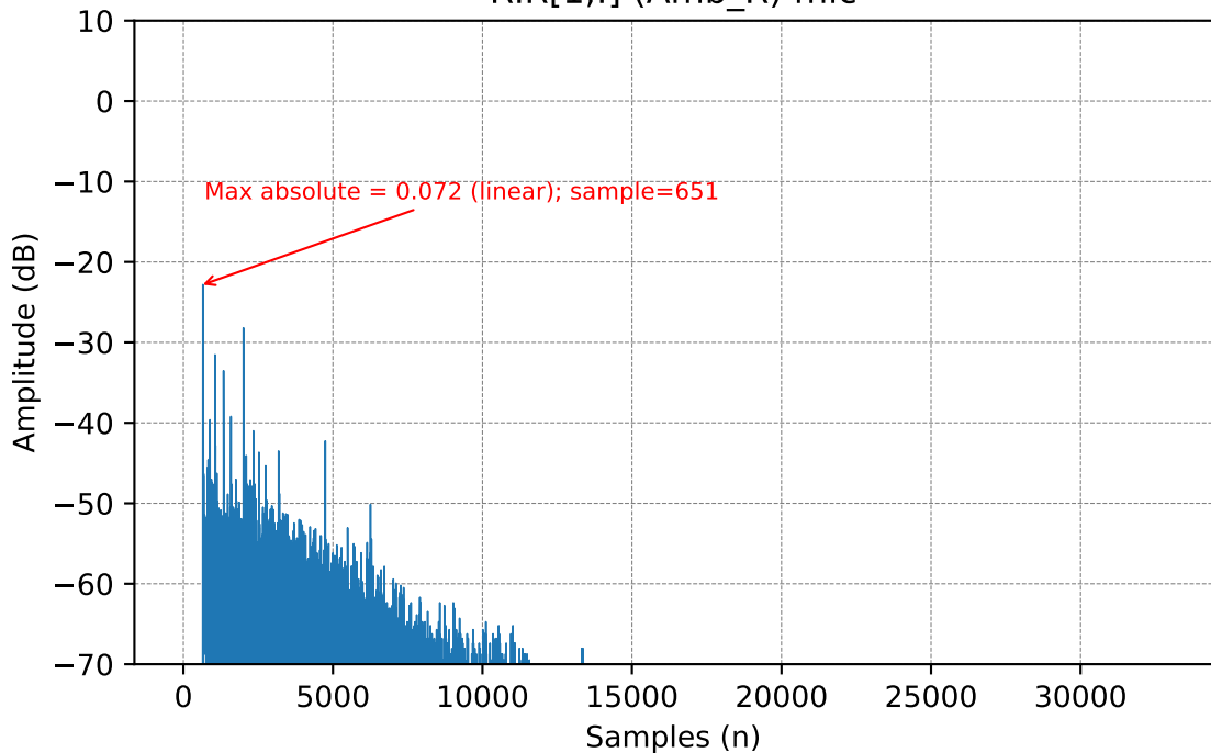
RIR[1,:] (Amb_R) mic
