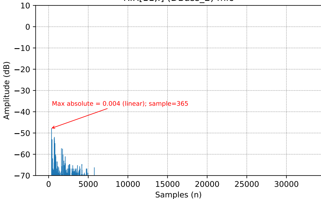
RIR[11,:] (DBass_2) mic
